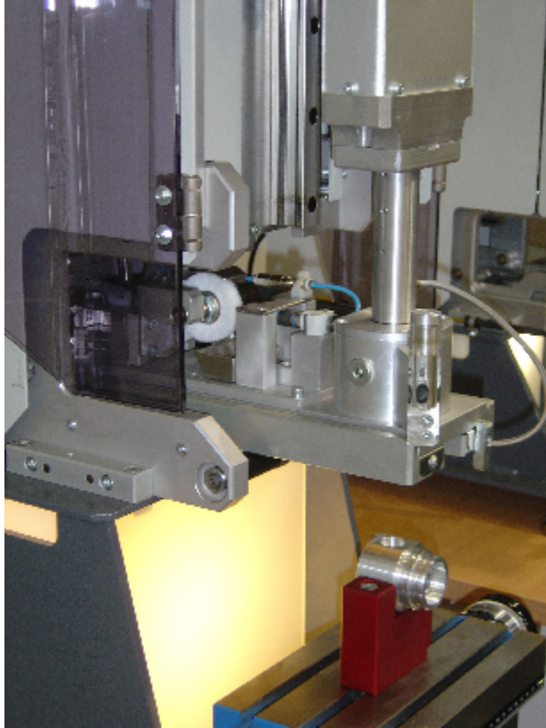
Druckdorn eingetaucht in das Mediumreservate.
